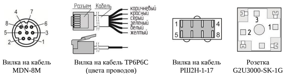
Рисунок Б.7 – Цоколевка разъемов кабелей.
