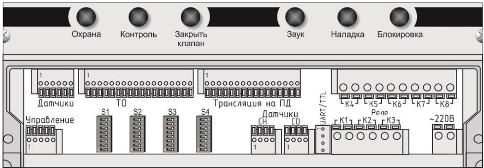
Рисунок 2 – Внешний вид клеммного отсека
