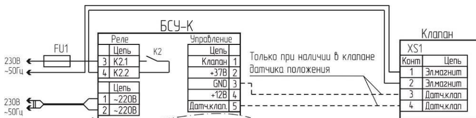
Рисунок Б.9 – Схема подключения клапана типа КПЭГ.
