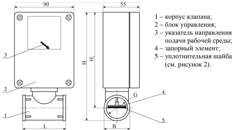
Рисунок 1 – Внешний вид клапана КЗЭДУГ.
