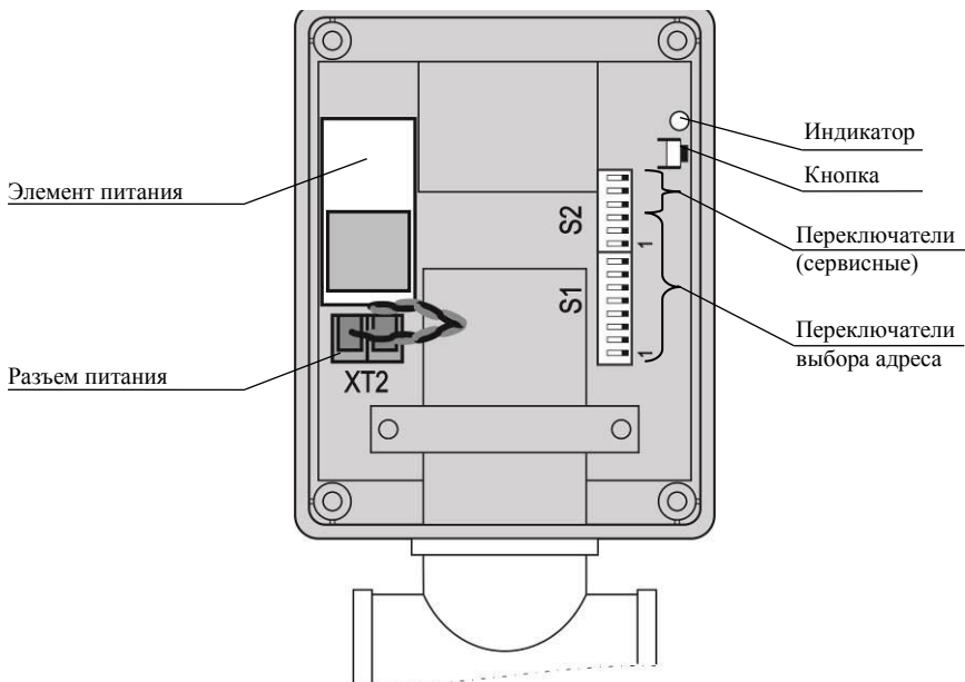
Рисунок 3 – Элементы управления.
