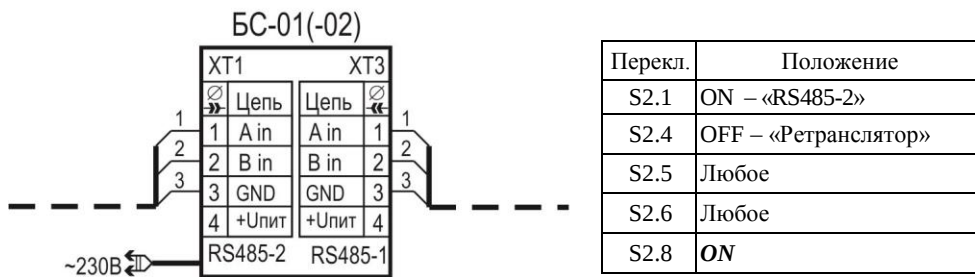
б) схема электрическая подключений
