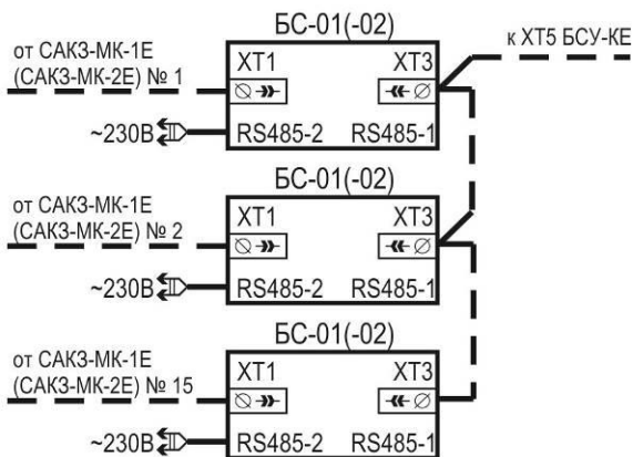
а) блок-схема
