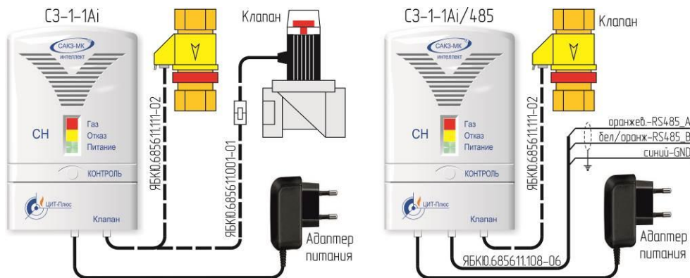
Рисунок Б.1 – Типовые схемы с клапаном (тип клапана показан условно)
