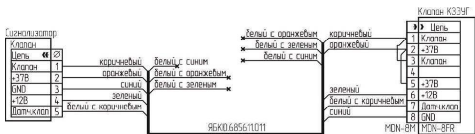
Рисунок В.5 – Схема подключения клапана КЗЭУГ с разъемом MDN8FR.
