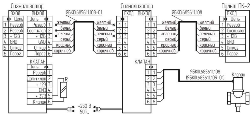
Рисунок В.7 – Схема соединений нескольких сигнализаторов с разъемами ТЛ1А-6Р6С с клапаном и пультом
