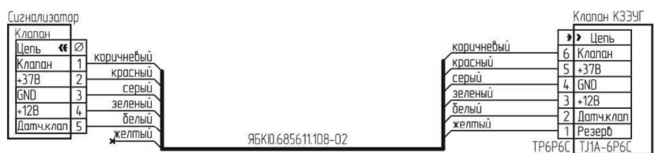
Рисунок В.6 – Схема подключения клапана КЗЭУГ с разъемом TJ1A-6P6C к сигнализатору с разъемами I5EDGLC-3,5
