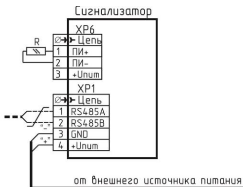
Рисунок Г.2 – Схема подачи питания для сигнализатора СЗ-2ЕВ
