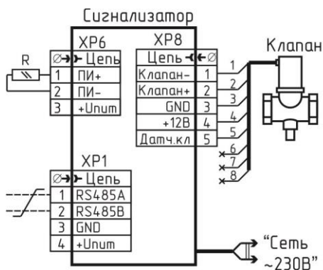
Рисунок Г.1 – Схема подключения клапана (кроме СЗ-2ЕВ)
