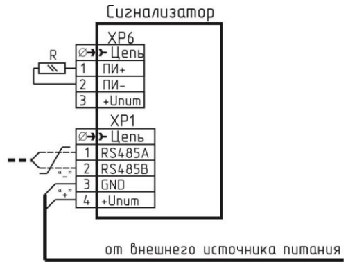
Рисунок Г.2 – Схема подключения питания сигнализатора С3-1ЕВ
