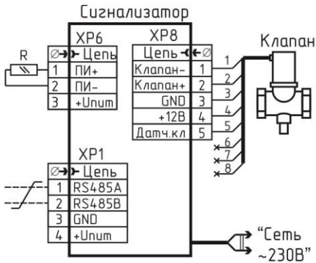
Рисунок Г.1 – Типовая схема подключения клапана (кроме С3-1ЕВ)
