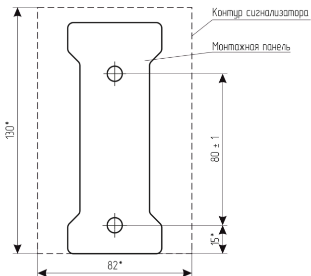
Рисунок В.1 – Монтажные размеры
