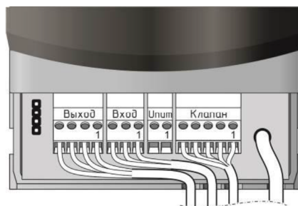
Рисунок 4 – Расположение разъемов
