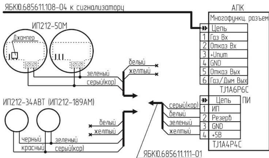
Рисунок 2 – Схема подключения пожарных извещателей
