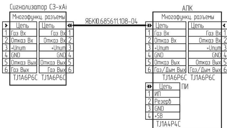
Рисунок 1 – Типовая схема подключения
