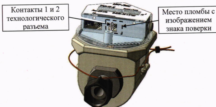
Рисунок 1 – Расположение контактов 1 и 2 технологического разъема
