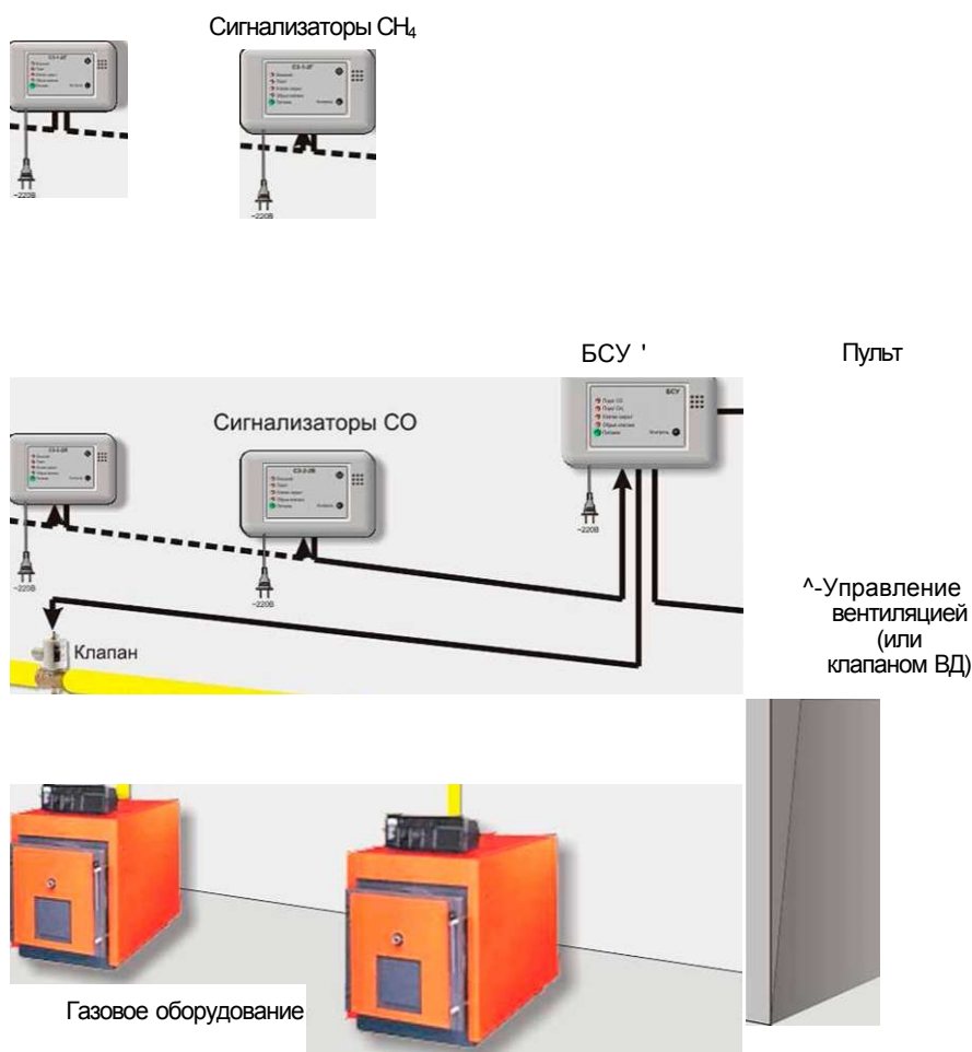
Система автоматического контроля загазованности САКЗ-МК-2. Типовая схема размещения
